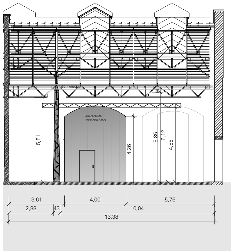
Querschnitt B-B'
