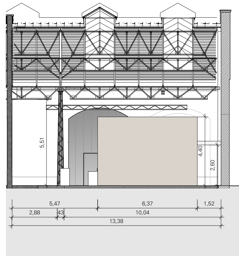
Querschnitt C-C'
